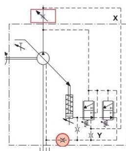
LS0 Load Sense
