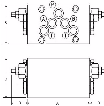
CETOP 5
