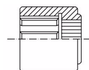
Splined Coupling MA 6x21x25 UNI 8953 A 22x19 DIN 5482 L=31
