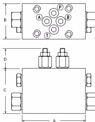
CETOP 3
