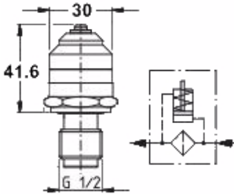
Pop Up Visual Indicator
