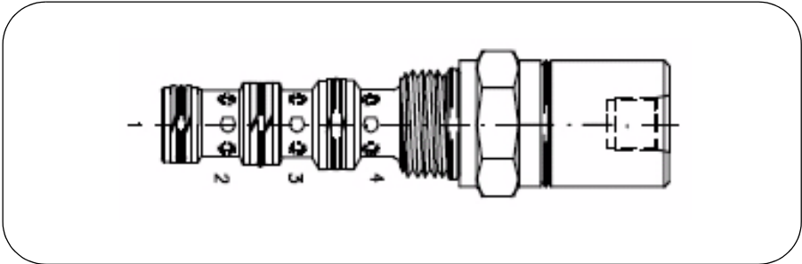
AODV
