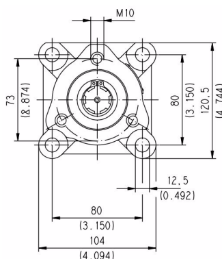
Splined Coupling MA 6x21x25 UNI 8953 A 22x19 DIN 5482 L=31
